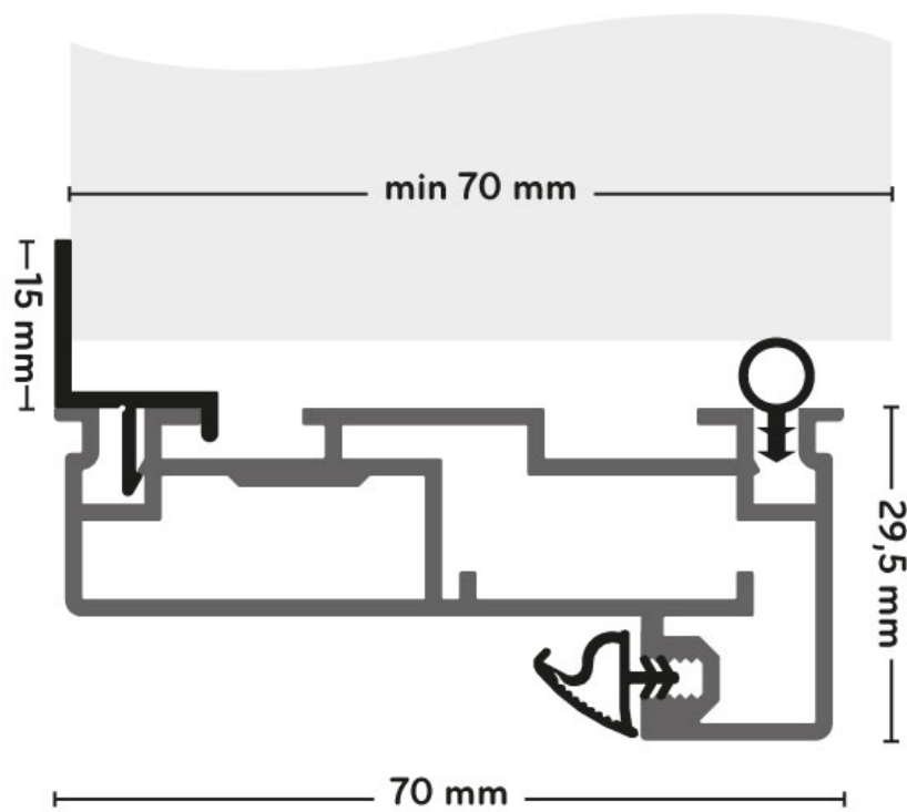
ALTEZZA ANTA LEAF HEIGHT
